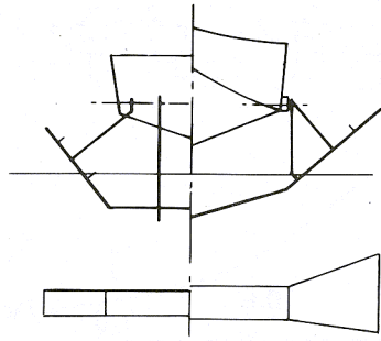
Figure 3.4.1 - Schertel-Sachsenberg Foil-System
