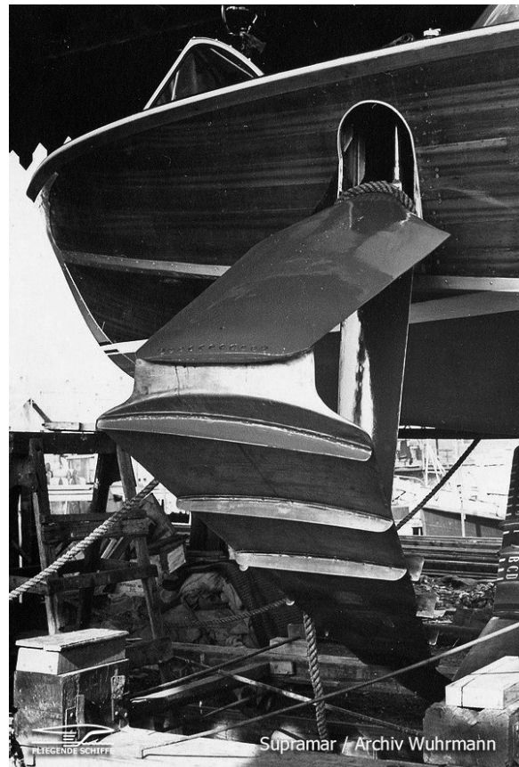
PT 10 Freccia D'Oro, Lake Lucerne, 1955
